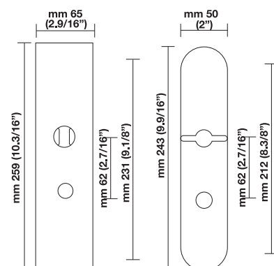
NES Narrow Plain Escutcheon
