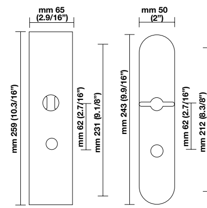
NES Narrow Plain Escutcheon
