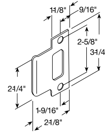
031471-001* Early Corbin Russwin single door
