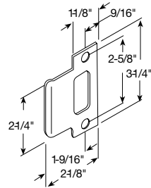
005164-000* ANSI Prep A115.2
