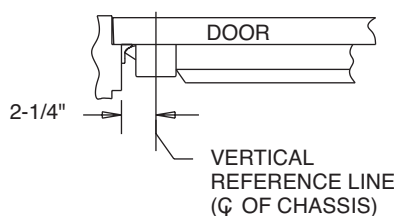
DOOR
